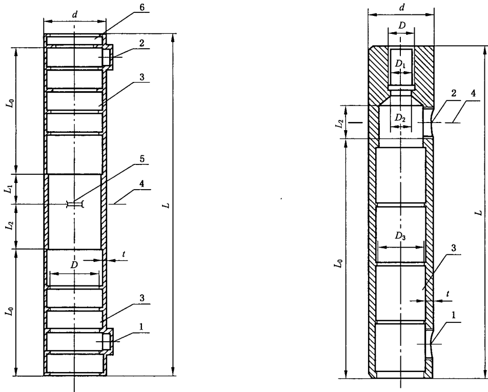
b) 半灌浆套筒
